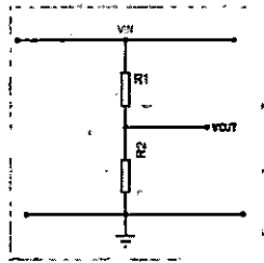
Gambar 10 : Pembagi tegangan
