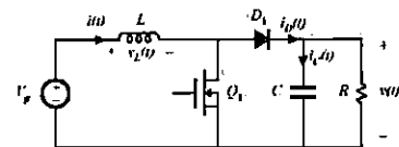
Gambar 1 : Topologi boost converter
