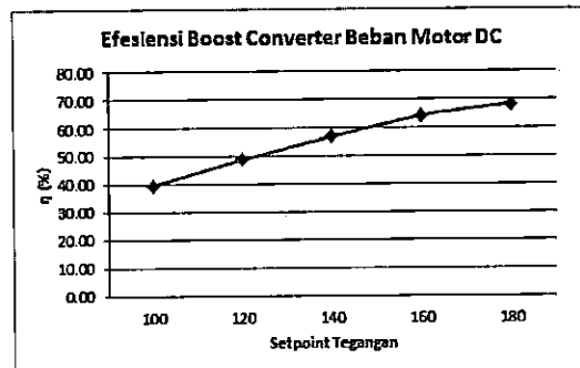
Gambar 46 : Grafik efisiensi boost converter beban motor DC
