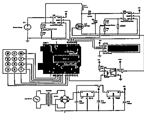
Gambar 25 : Rangkaian Keseluruhan
