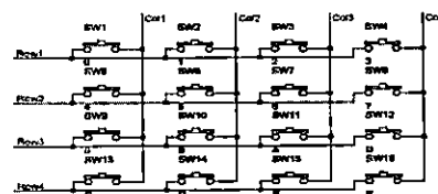
Gambar 8 : Konstruksi Matrix Keypad 4x4 Untuk Mikrokontroler.
