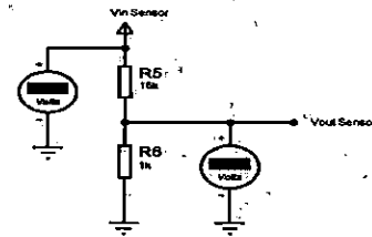
Gambar 39 : Rangkaian pengujian sensor tegangan
