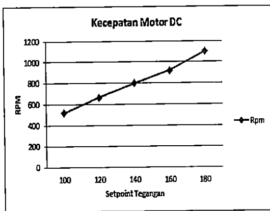
Gambar 44 : grafik kecepatan motor DC
