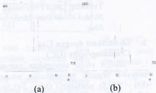
Gambar 3. Kromatogram Methylene Blue (a) Sebelum Proses Degradasi Dan (B) Sesudah Proses Degradasi
