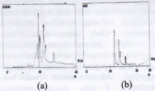
Gambar 3. Kromatogram Methyl Violet (a) sebelum proses degradasi dan (b) sesudah proses degradasi
