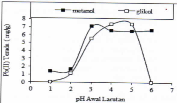
Gambar 3. Pengaruh pH larutan terhadap biosorpsi biomassa yang diperlakukan dengan reagen pemodifikasi gugus fungsi
