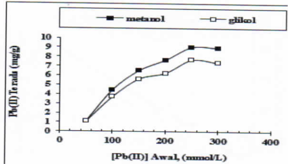
Gambar 4. Pengaruh konsentrasi larutan ion logam terhadap daya serap biomassa termodifikasi gugus karboksilat dibandingkan dengan daya serap biomassa murni
