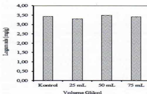
Gambar 2. Pengaruh volume pemodifikasi pemodifikasi gugus fungsi karbonil terhadap serapan biomassa alga hijau S. subsalsa
