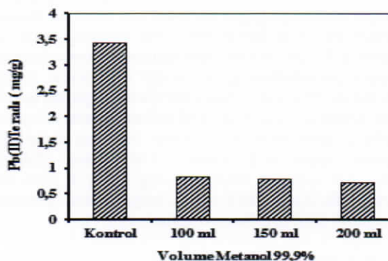
Gambar 1. Pengaruh volume pemodifikasi gugus karboksil terhadap kapasitas serapan biomassa alga hijau S. subsalsa
