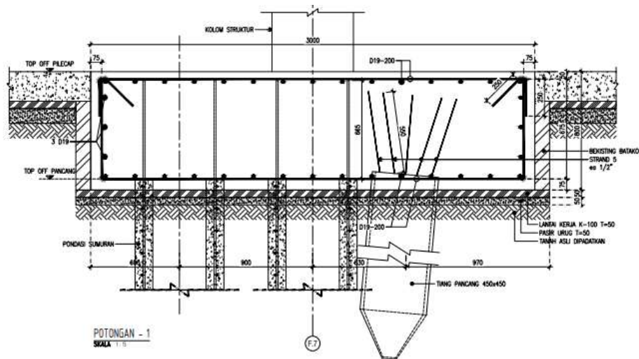
Gambar 4. Potongan Fondasi (Sumber : Dokumen PT-X, 2021)
