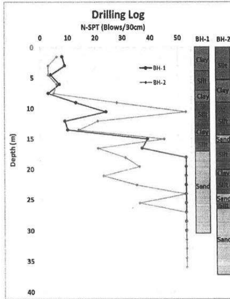
Gambar 1. Profil N_{SPT} versus depth (Sumber : Dokumen PT-X, 2021)
