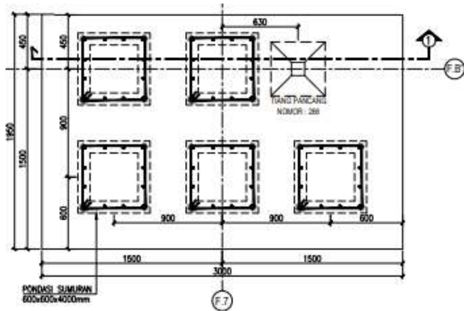
Gambar 3. Denah Perletakan Sumuran (Sumber : Dokumen PT-X, 2021)
