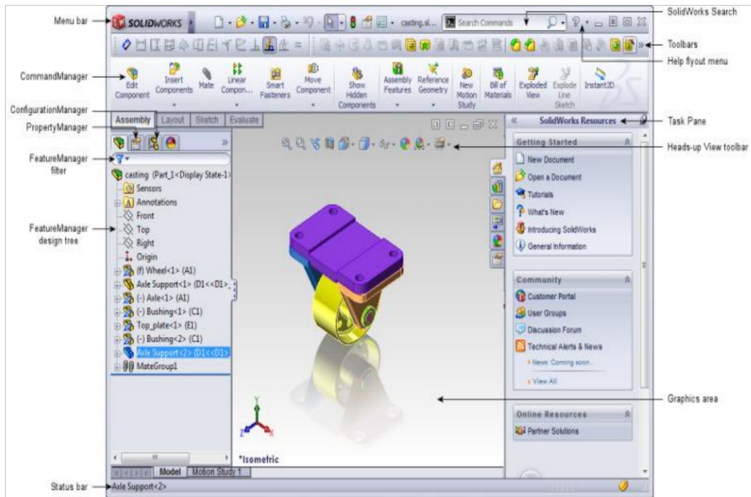
Gambar 4.15 Komponen Solidwork
