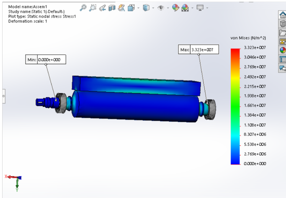
Gambar 5.2 Hasil simulasi solidwork pada bearing dengan pemberian force sebesar 248.430 N
