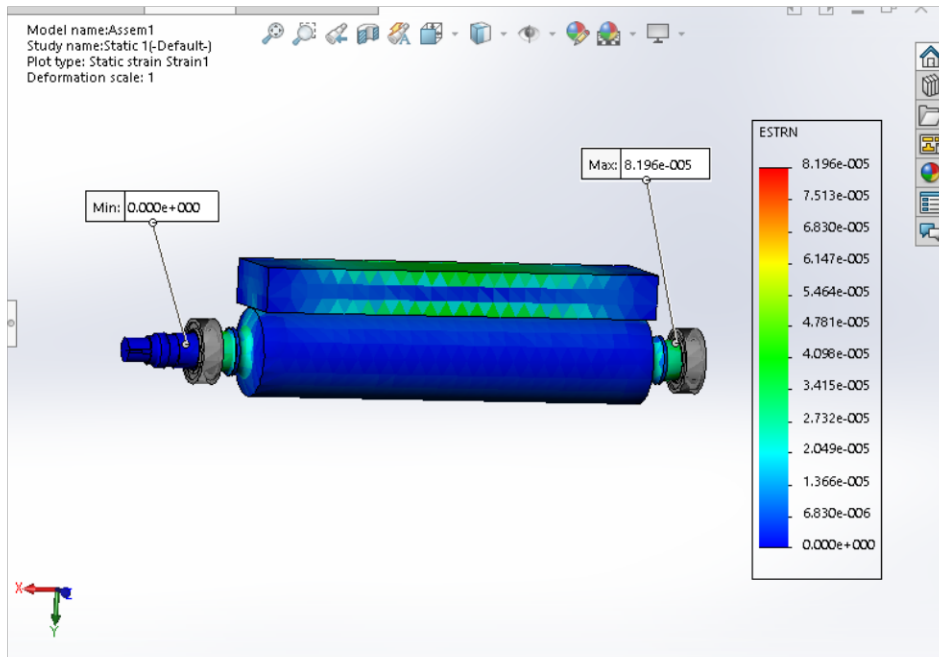
Gambar 5.4 Hasil simulasi equivalent pada bearing dengan load 25 ton
