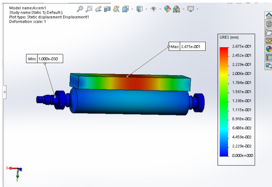
Gambar 5.3 Hasil simulasi displacement pada bearing dengan load 25 ton
