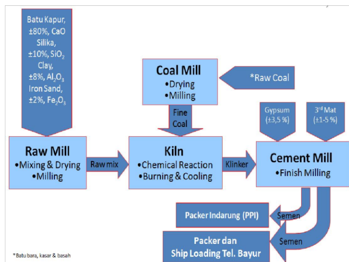
Gambar 3.3 Diagram Aliran Proses Pembuatan Semen
