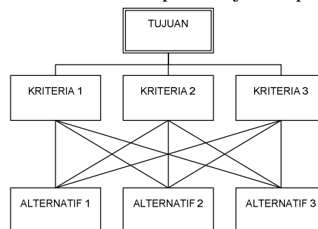
Gambar 1. Struktur hirarki
