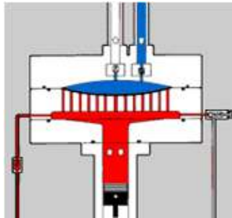
Gambar 4.3 Kompresor diafragma
