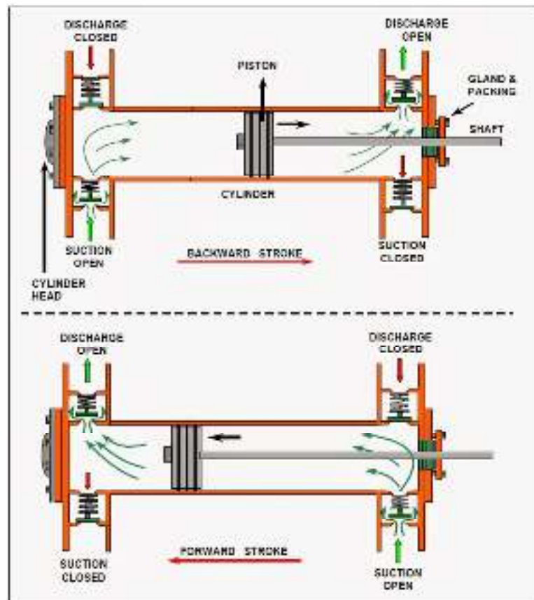
Gambar 4.2 Kompresor piston kerja ganda
