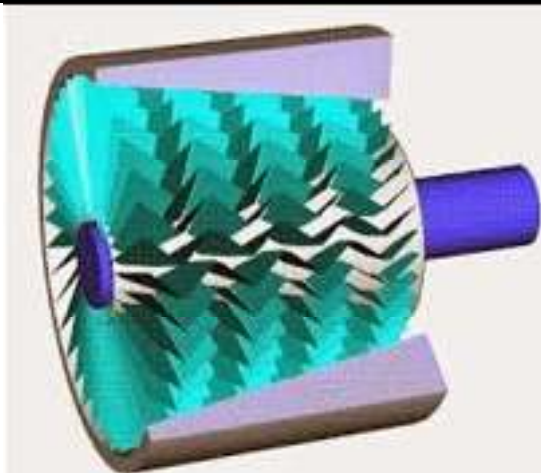
Gambar 4.6 Kompresor aksial
