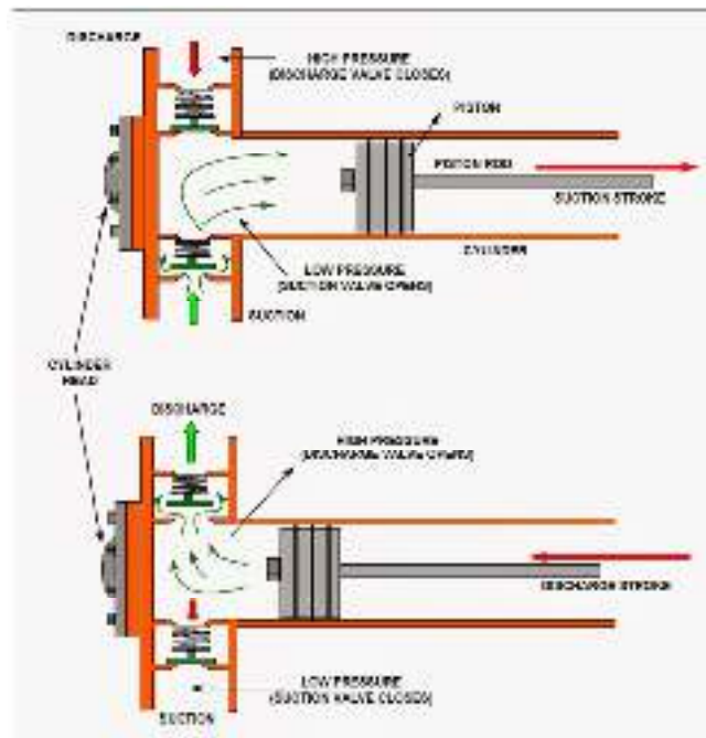
Gambar 4.1 kompresor piston kerja tunggal
