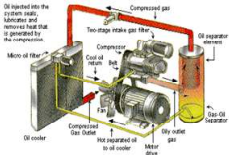
Gambar 4.4 Kompresor screw
