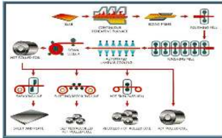
Gambar 2.10 Alur Proses produksi HSM
