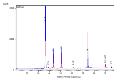
Gambar 2 : Hasil XRD
