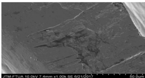
Gambar 3 : Sebelum kalsinasi
