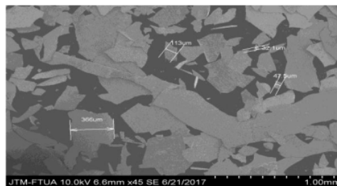
Gambar 4 : Setelah Kalsinasi
