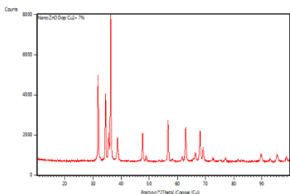
Gambar 1. Difraktogram nano ZnO doping Cu 7%.
