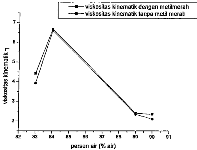
Gambar 55. Perbandingan viskositas kinematik sistem SDS, Pentanol dan Air pH=4,5 fasa L 2 dengan dan tanpa keberadaan metil merah
