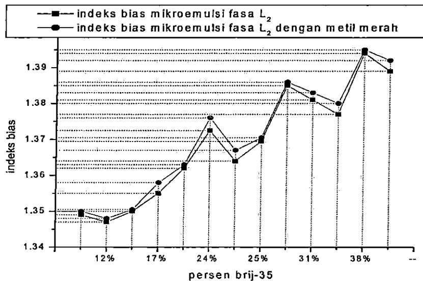
Gambar 41. Indeks bias mikroemulsi sistem air (pH=4,5), brij-35 dan pentanol fasa L 1 dengan metil merah dan tanpa metil merah
