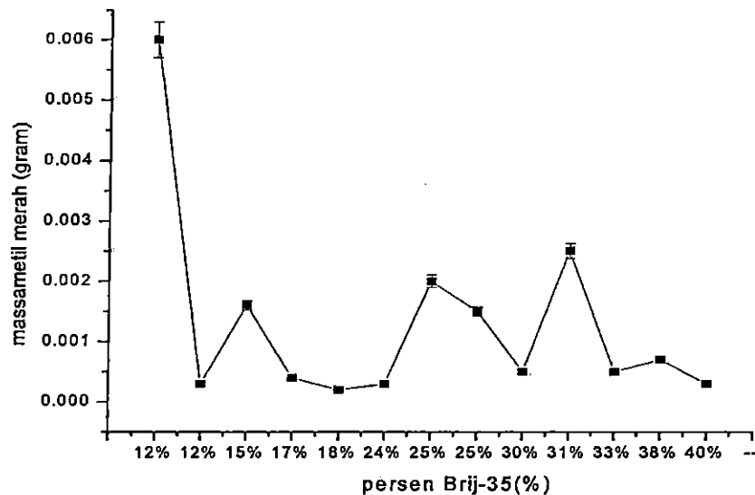
Gambar 33. Solubilitas metil merah terhadap prosentase brij-35 pada fasa L 2 sistem Air pada pH=4,5, Brij-35, dan Pentanol
