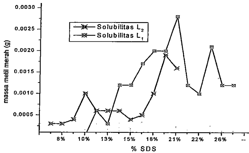
Gambar 16. Solubilitas metil merah dalam fasa L 1 dan L 2 sistem air (pH=4,5), SDS dan pentanol
