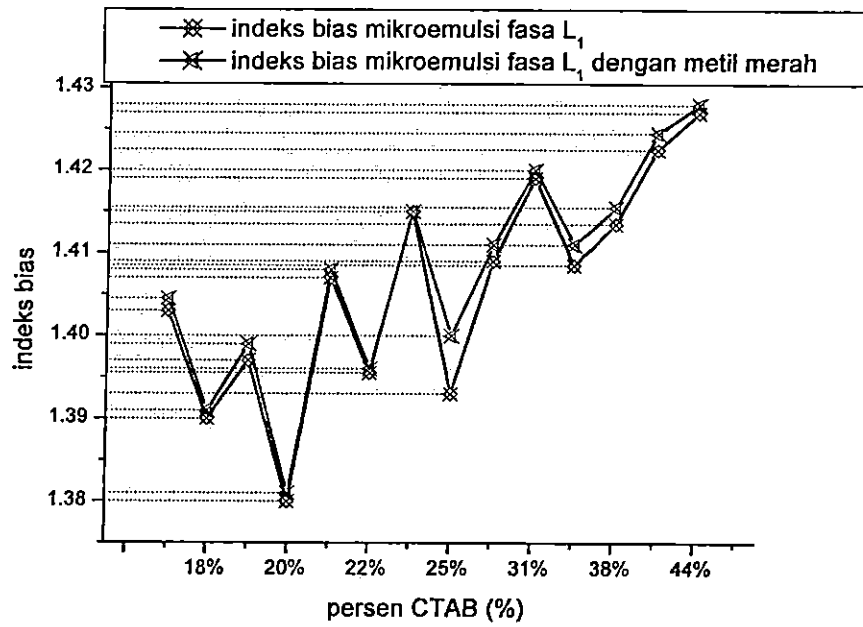
Gambar 38. Indeks bias mikroemulsi sistem air (pH=4,5), CTAB dan pentanol fasa L 1 dengan metil merah dan tanpa metil merah
