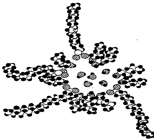
Gambar 5. Representasi misel inversi dalam pelarut organik jenuh
