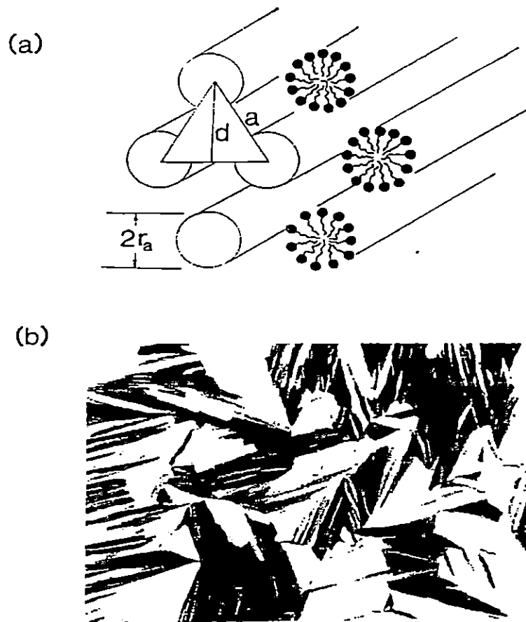
Gambar 8. (a) Representasi skematis model kristal cair heksagonal, dan (b) pola optik nongeometriskristal cair heksagonal.
