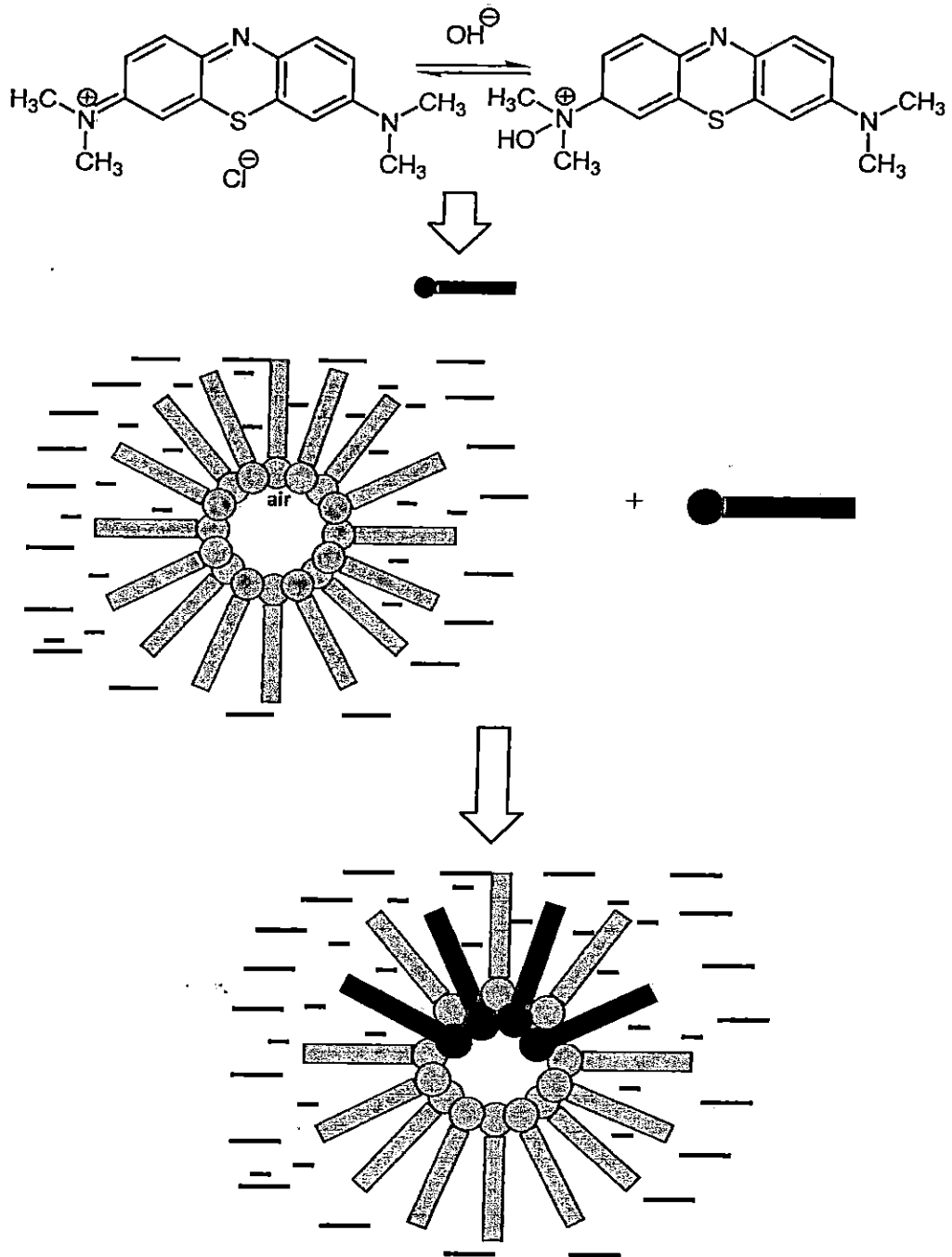
Gambar 23. Mekanisme solubilitas metil biru dalam fasa L 1
