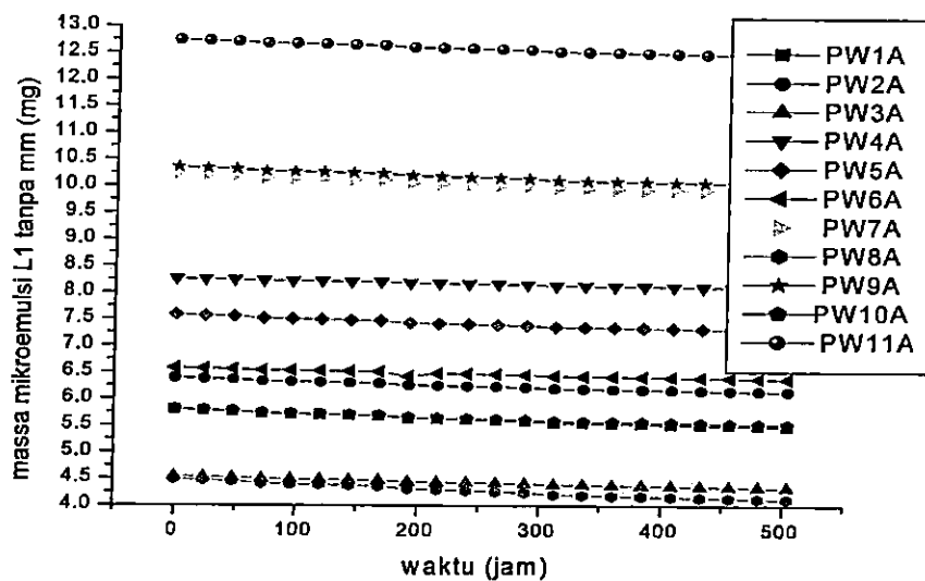
Gambar 44. Tren laju penguapan sistem SDS, Pentanol dan Air pH=4,5 fasa L_1
