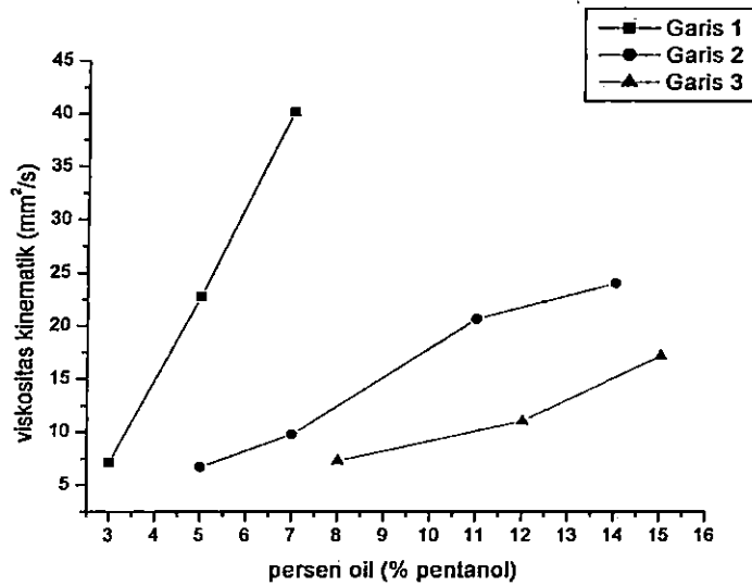
Gambar 63. Perbandingan viskositas kinematik sistem Brij-35, Pentanol dan Air pH=4,5 fasa L 2 dengan dan tanpa keberadaan metil merah
