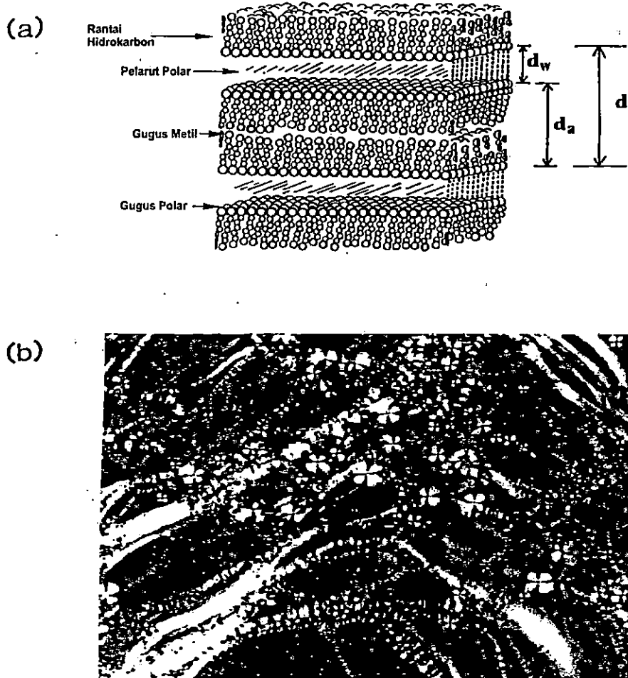
Gambar 7. (a) Representasi kristal cair lamelar ( d : jarak perulangan; d_a dan d_w : ketebalan amfifil dan lapisan air); (b) pola optik kristal cair lamelar.
