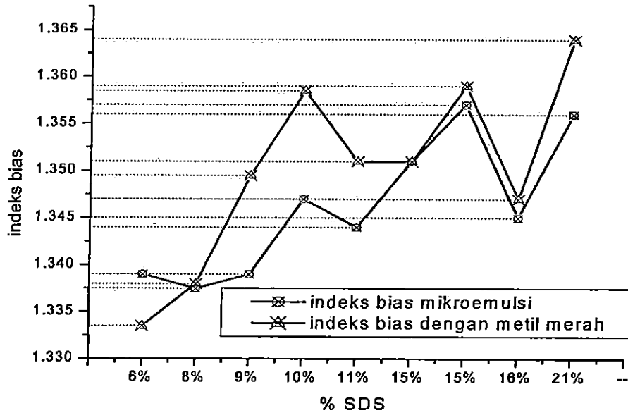
Gambar 37. Indeks bias mikroemulsi sistem air (pH=4,5), SDS dan pentanol fasa L 2 dengan metil merah dan tanpa metil merah
