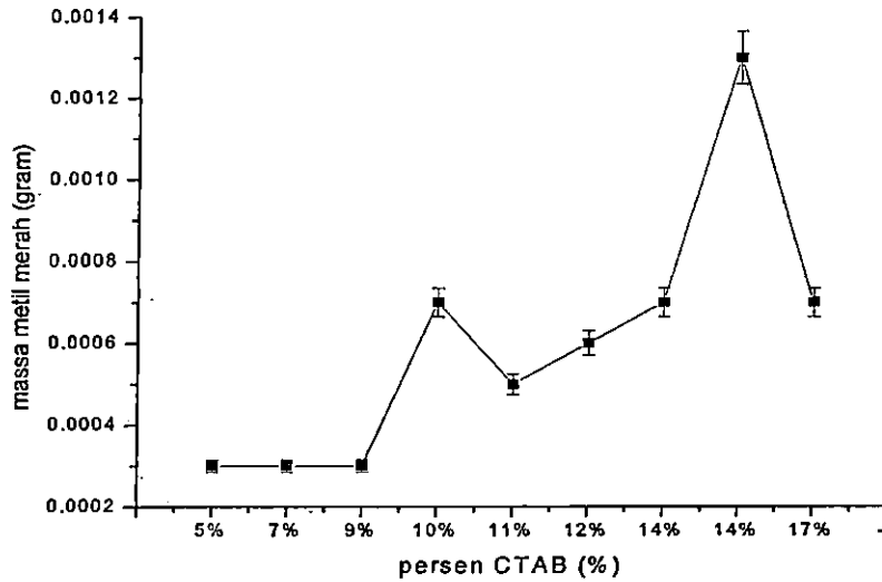
Gambar 27. Solubilitas metil merah terhadap prosentase CTAB pada fasa L 2 sistem Air pH=4,5, CTAB, dan Pentanol
