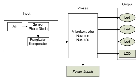
Gambar 7 Blok Diagram Rangkaian
