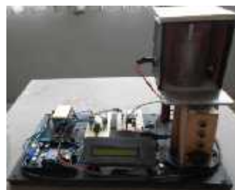
Gambar 9 Gambar Alat Tampak Depan
