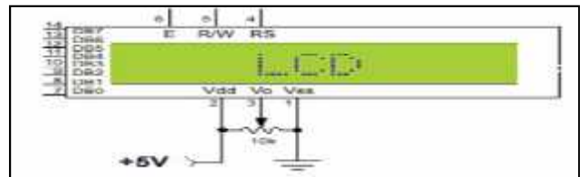
Gambar 4 Rangkaian LCD
