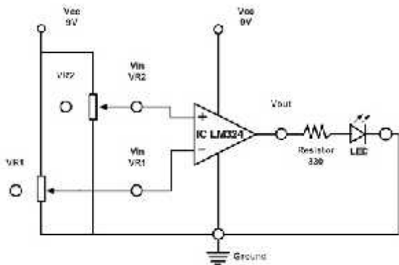
Gambar 2 Rangkaian komparator
