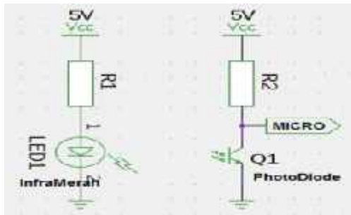
Gambar 1. Gambar Rangkaian Sensor.
