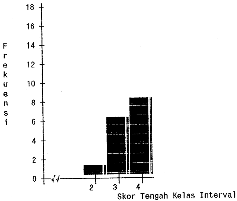
HISTOGRAM INTENSITAS WARNA DG DAUN MANGGA GELUPAN 10 KALI
