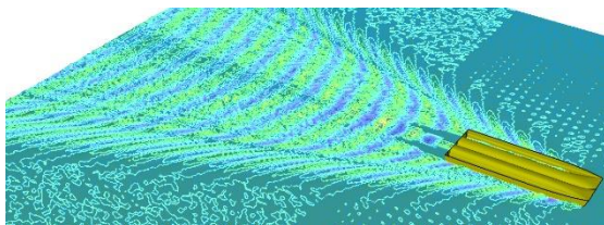
Gambar 3. Hasil simulasi layar kapal dengan Maxsurf
