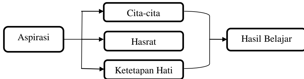
Gambar 1. Kerangka Konseptual
